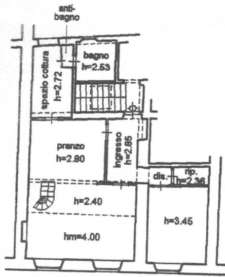
PIANO TERZO
